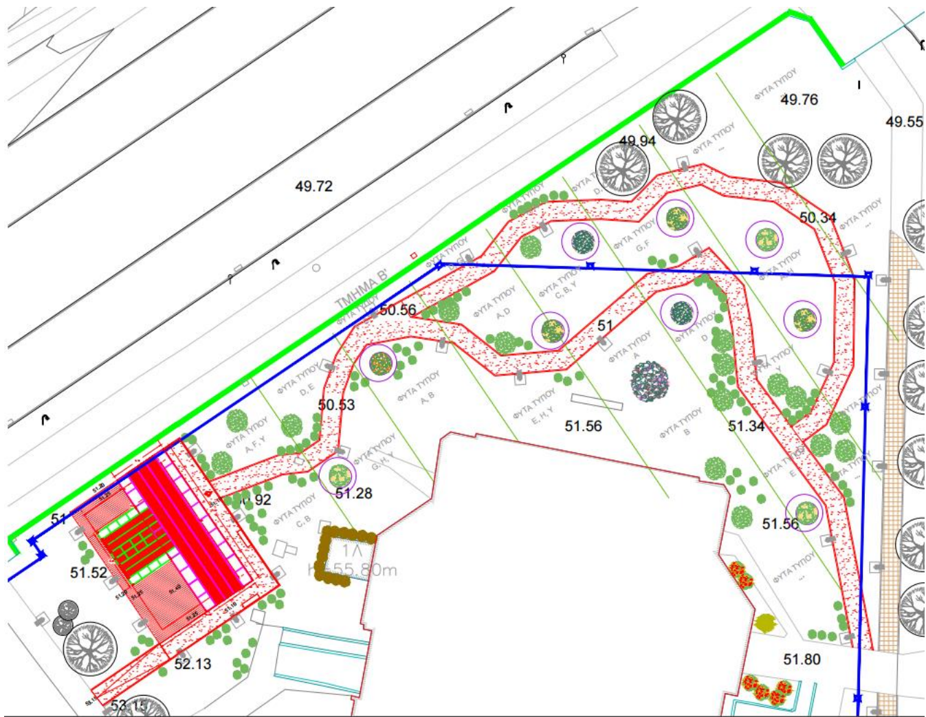
Εικόνα 7. Κάτοψη της διαμόρφωσης μονοπατιών με δάπεδο κουρασάνι περιμετρικά του Συνεδριακού
