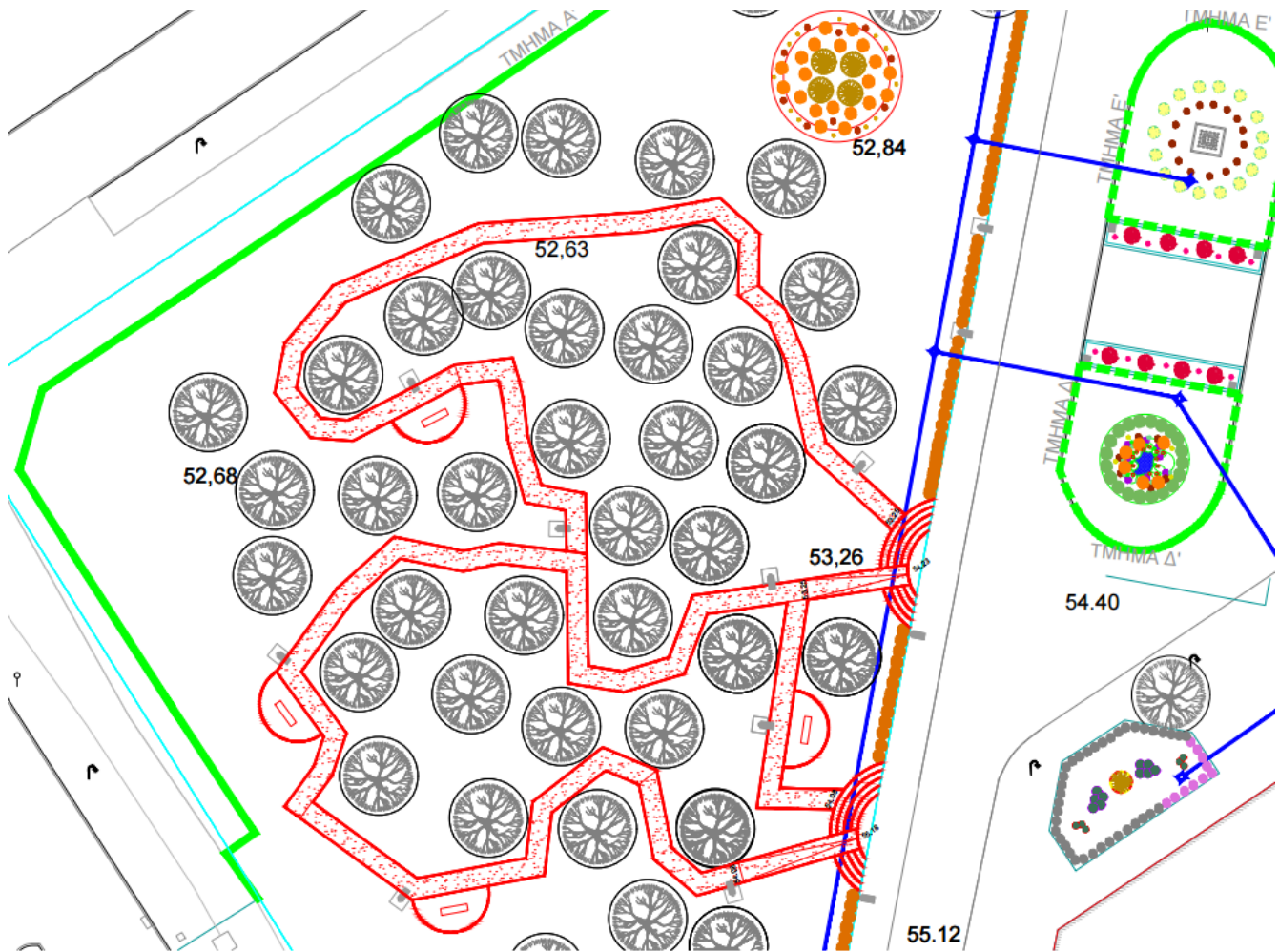
Εικόνα 5. Κάτοψη διαμόρφωσης μονοπατιών στον Ελαιώνα
