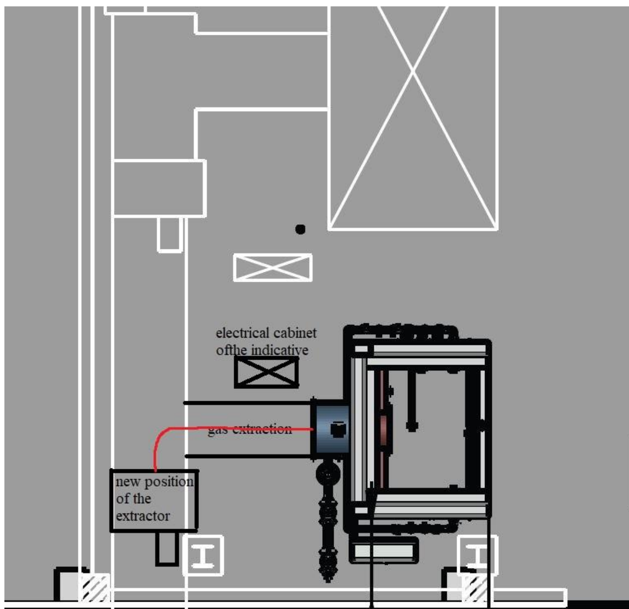
Σχέδιο 1. Σχηματική απεικόνιση του υπάρχοντος συστήματος απαγωγής καυσαερίων στο οποίο θα πρέπει να πραγματοποιηθεί η προσαρμογή του συστήματος του νέου κλιβάνου.
